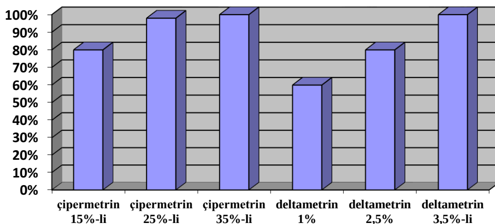
Şək. 5. İnsektisidlərə qarşı hünülərin həssaslığı
