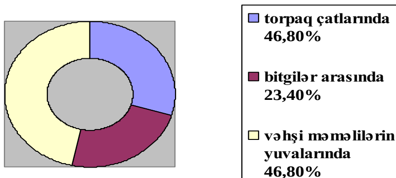
Şək. 3. Tərtər rayonunda təbii ocaqlarda hünülərin say intensivliyi
