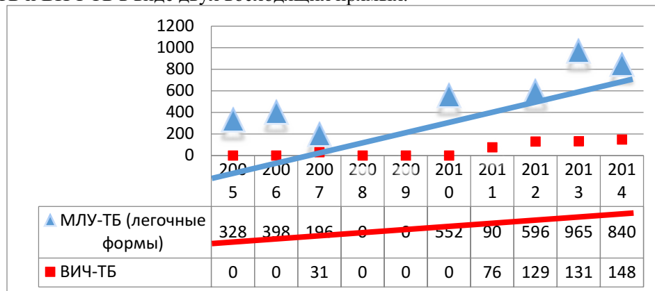
Рис.3. Динамика ТБ/ВИЧ-инфекции и легочных форм МЛУ/ШЛУ-ТБ за последнее десятилетие в Азербайджане
