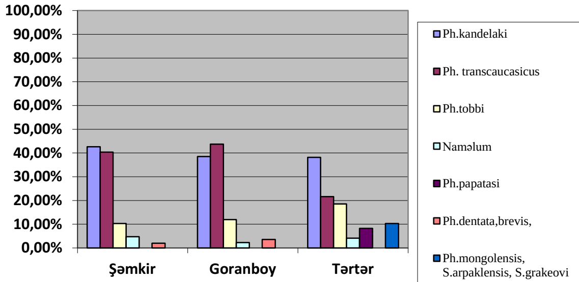
Şək. 4. Şəmkir, Goranboy, Tərtər rayonlarında epidemioloji cəhətdən təhlükəli hünülərin növ intensivliyi
